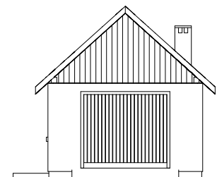
ELEWACJA FRONTOWA
