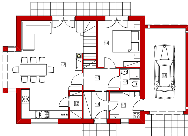
RZUT PARTERU
