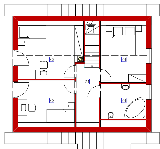
RZUT PODDASZA
